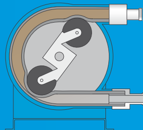
Нагнетательная сторона
